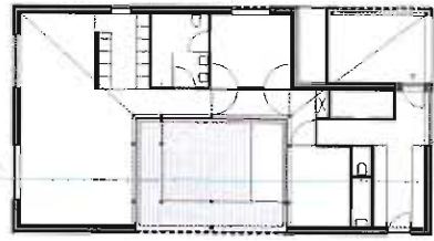
Livello 1 / Level 1
