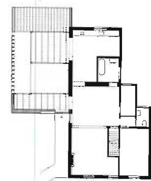
Livello 1 / Level 1
