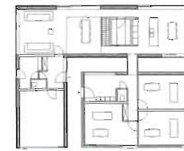
Livello 1 / Level 1
