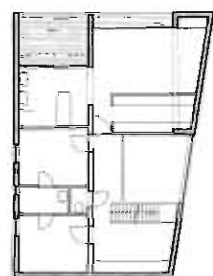
Livello 2 / Level 2
