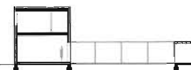
Sezione / Section
